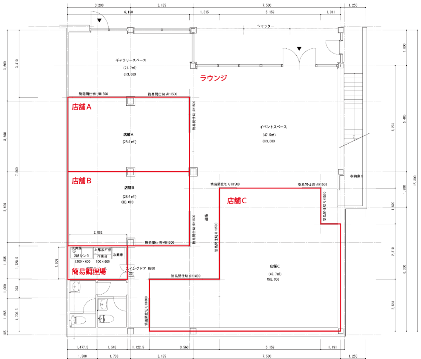
別図「吉沼まちかどテラス平面図」
